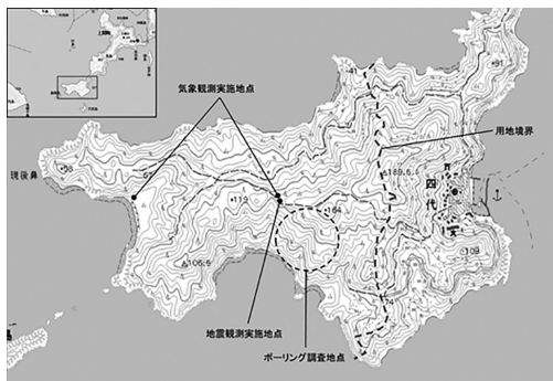
ボーリング調査地点 (提供 中国電力)
