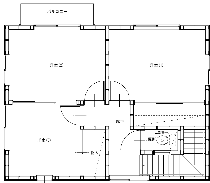
2階平面図
