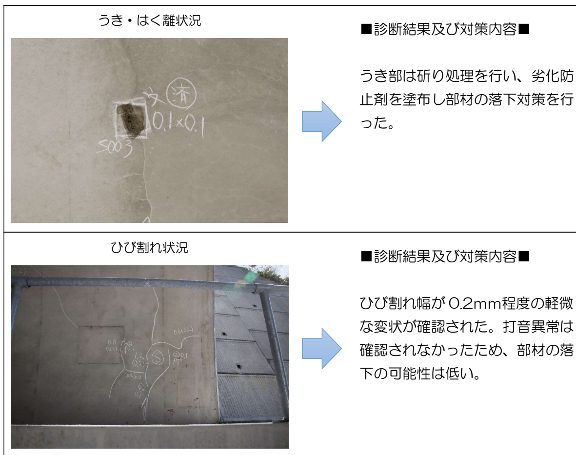
写真 2-3 トンネル変状事例
